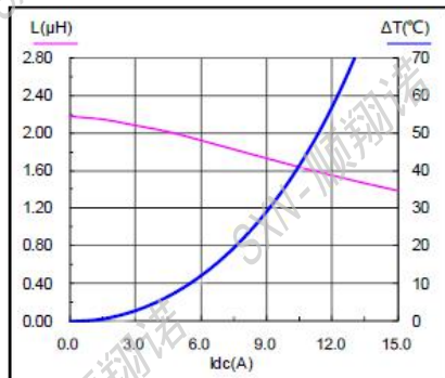
SMMS0650-2R2M
